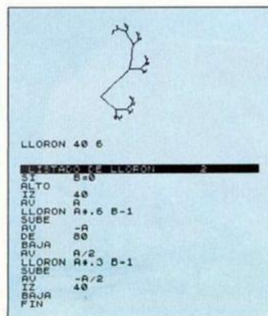
Procedimiento LLORON. Parámetro 40 6.
